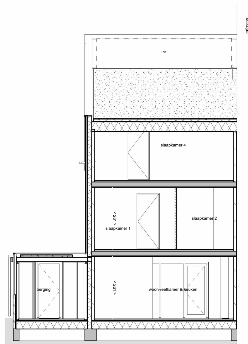
doorsnede A
