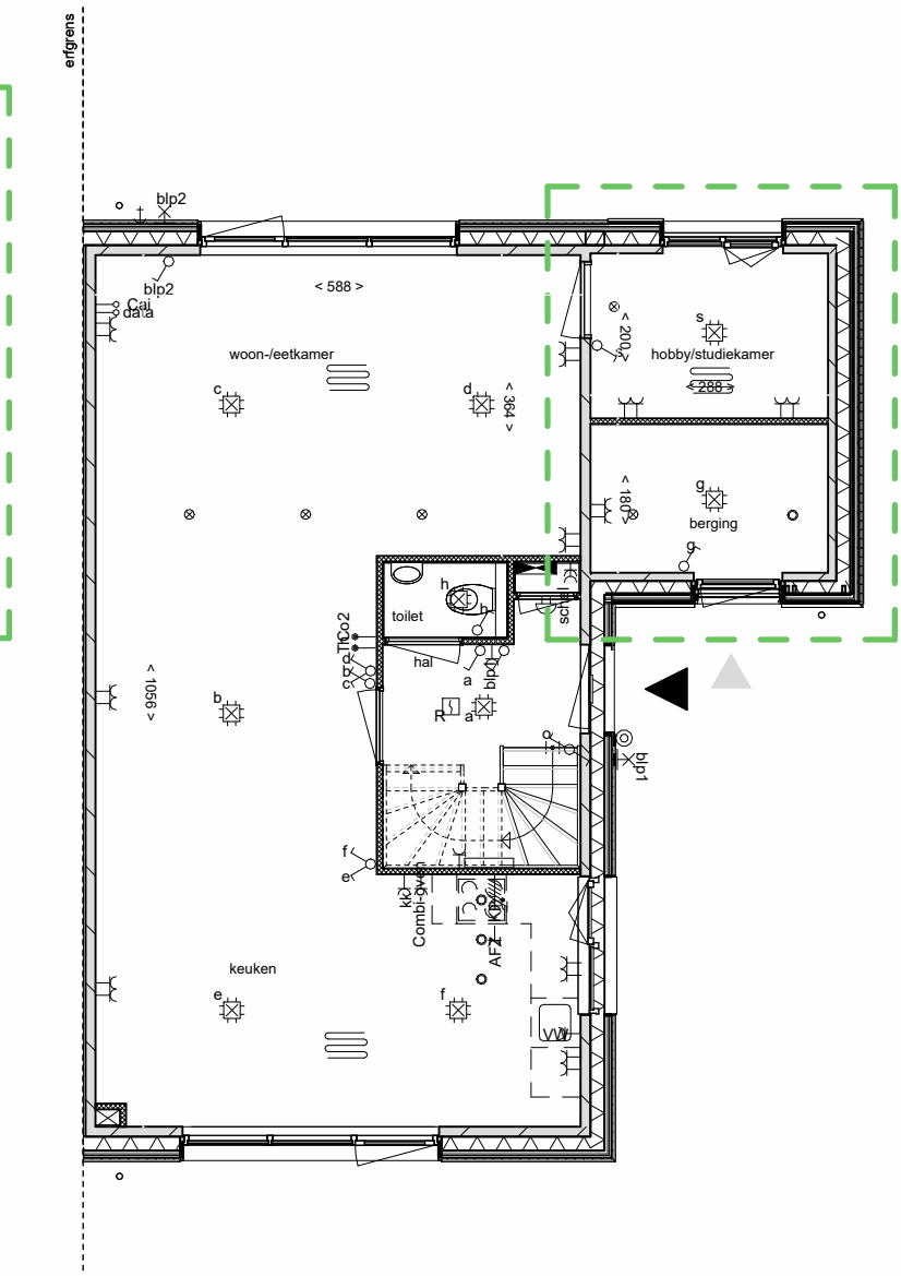
begane grond
