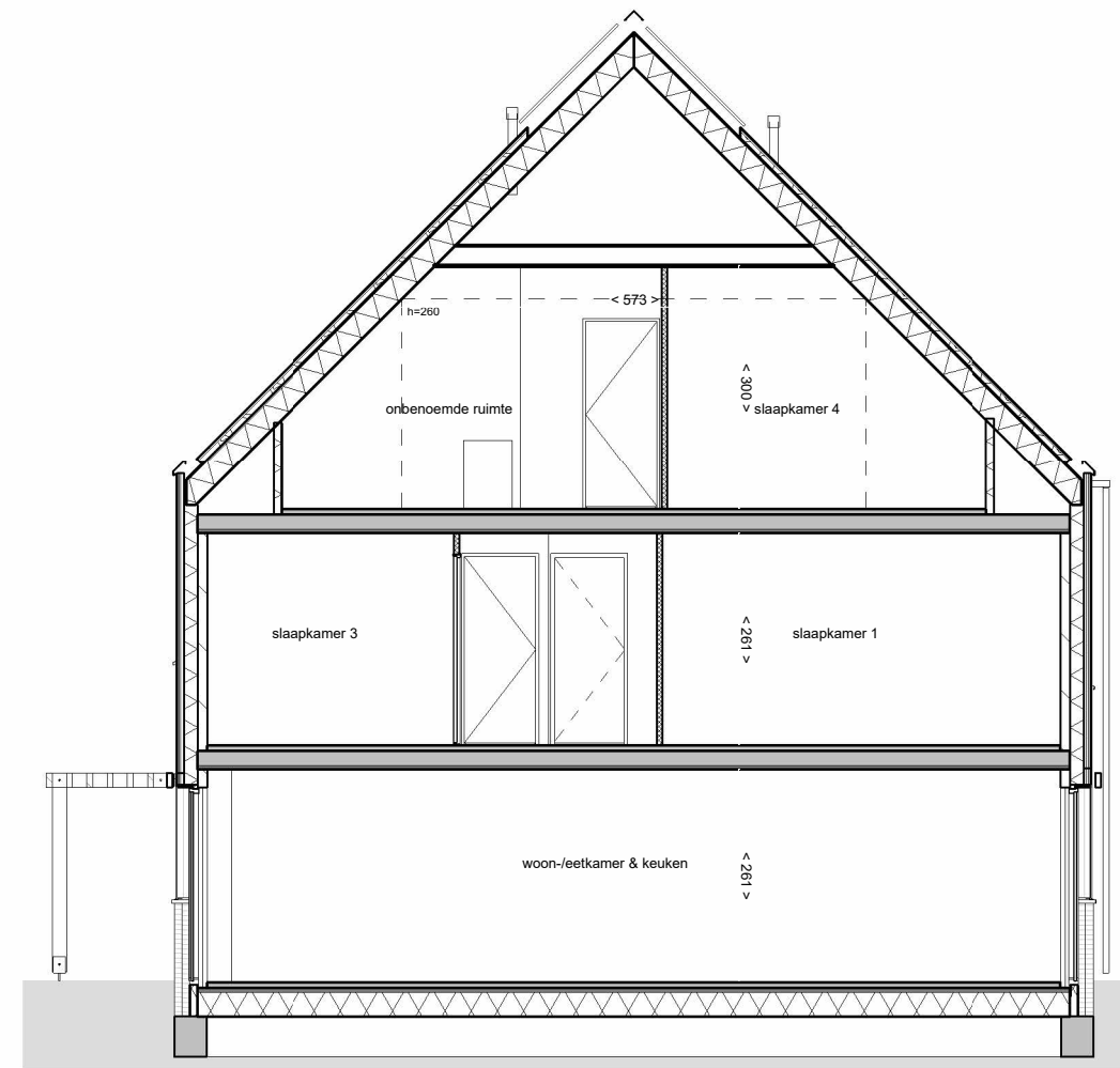
doorsnede B
