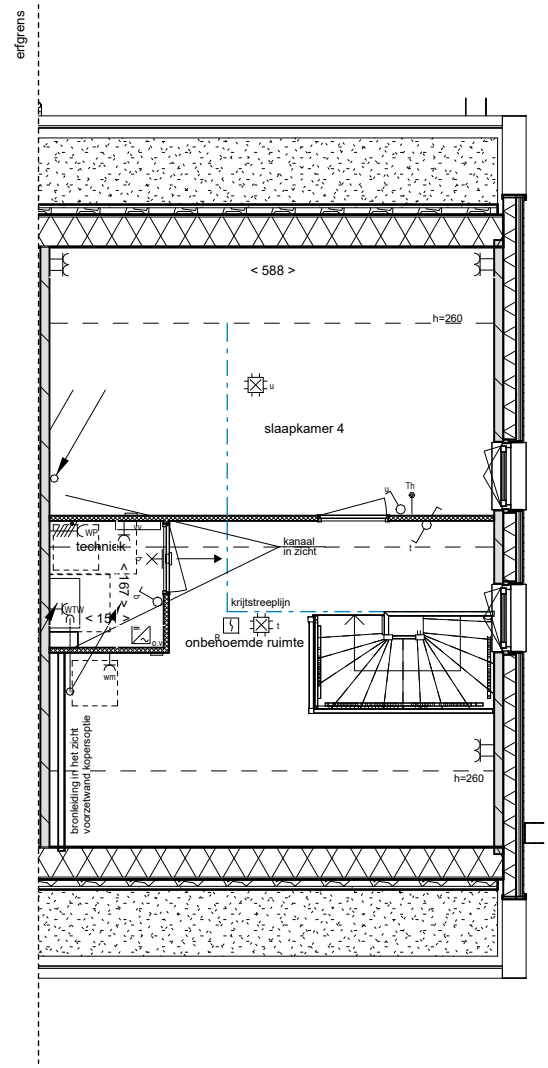
02 tweede verdieping
