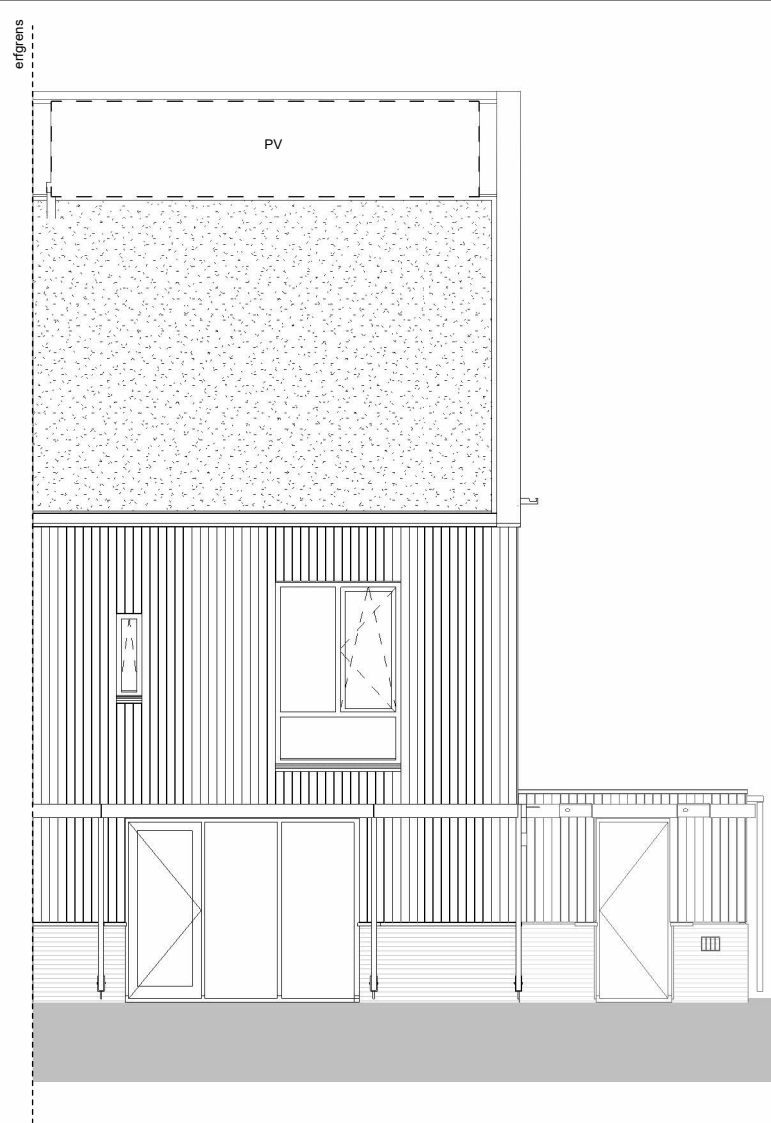
OV - 2k-XL - VK - bnr.105 - voorgevel
