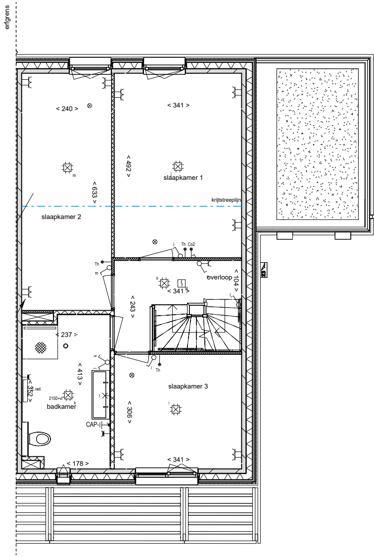
01 eerste verdieping
