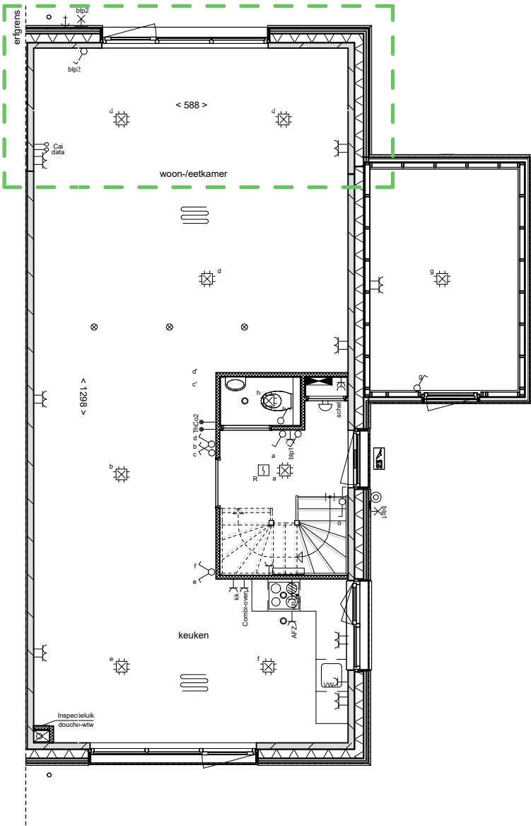
begane grond
