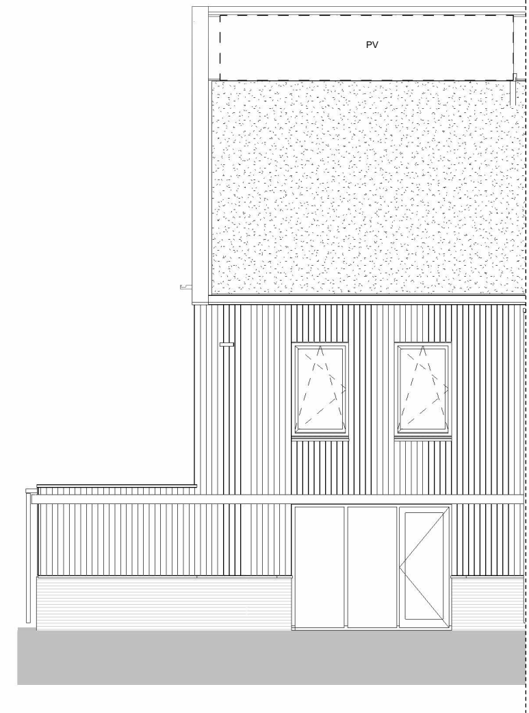
OV - 2k-XL - VK - bnr.105 - achtergevel
