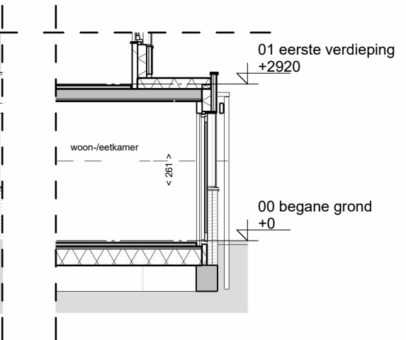
code 10110 / 20: uitbouw achtergevel 120cm
